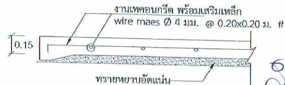
แบบขยาย GS2
