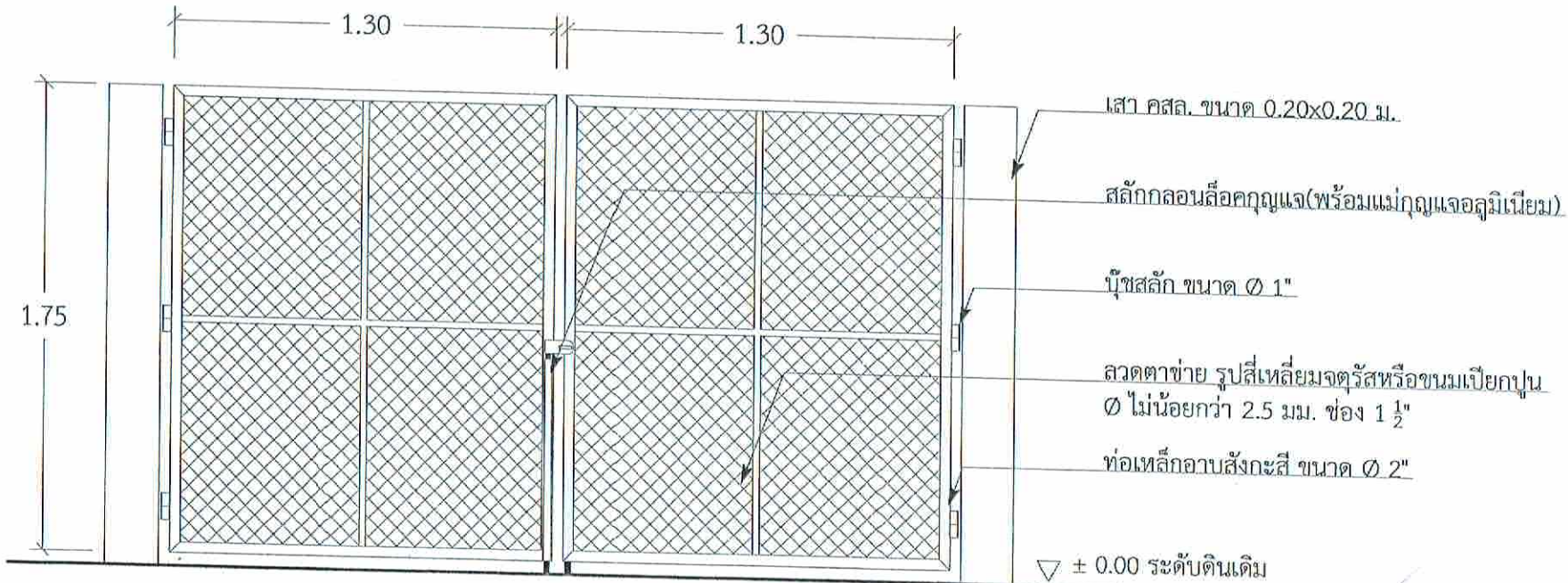
รูปด้านหน้า(ประตูรั้ว)
