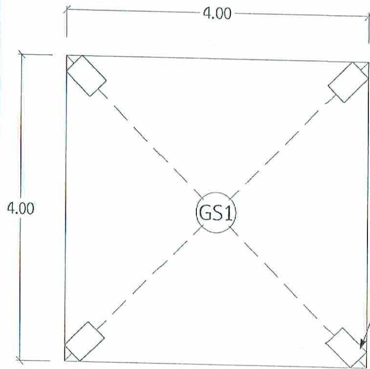
แปลนเทพื้น คสล. จุดที่ 3 (ใต้หอถังสูง)
