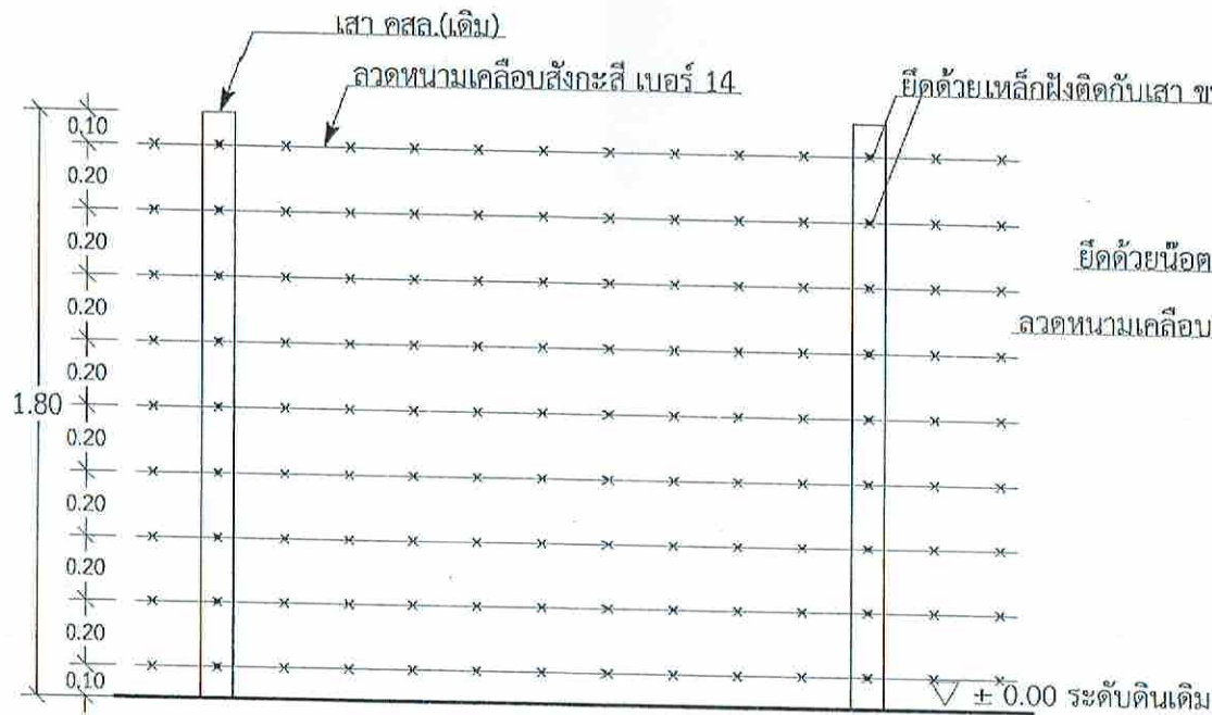
รูปด้าน(รื้อลวดหนาม)
