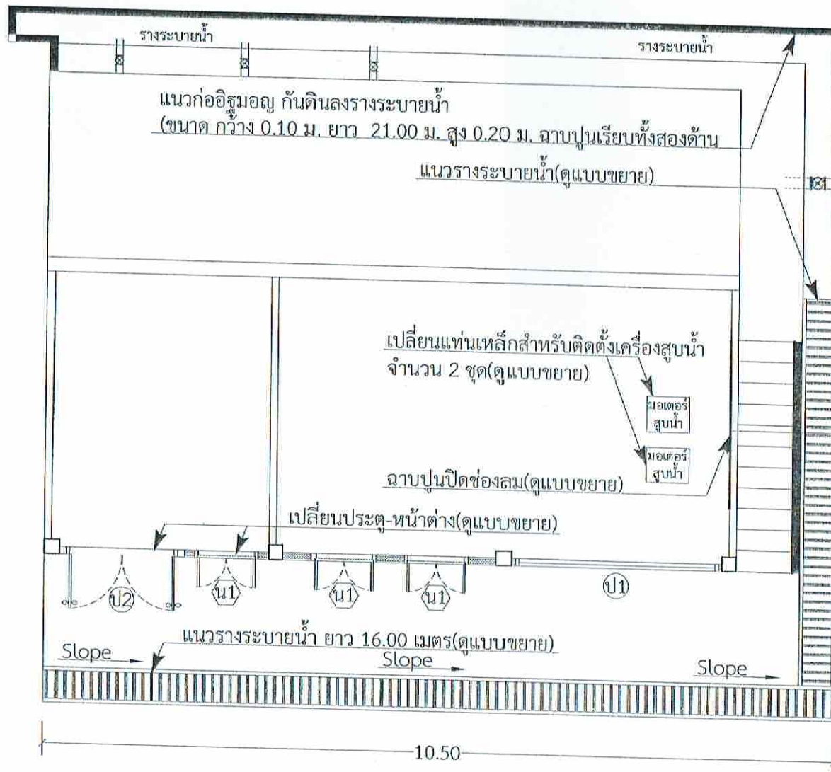
แบบผังบริเวณ อาคารผลิตน้ำประปา หมู่ที่ 7
