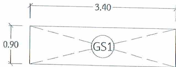
แปลนเทพื้น คสล. จุดที่ 5 (ใต้บันไดขึ้นโรงกรอง)
