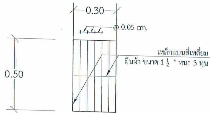
แปลนแสดงการเสริมเหล็กลูกนอนบันได
